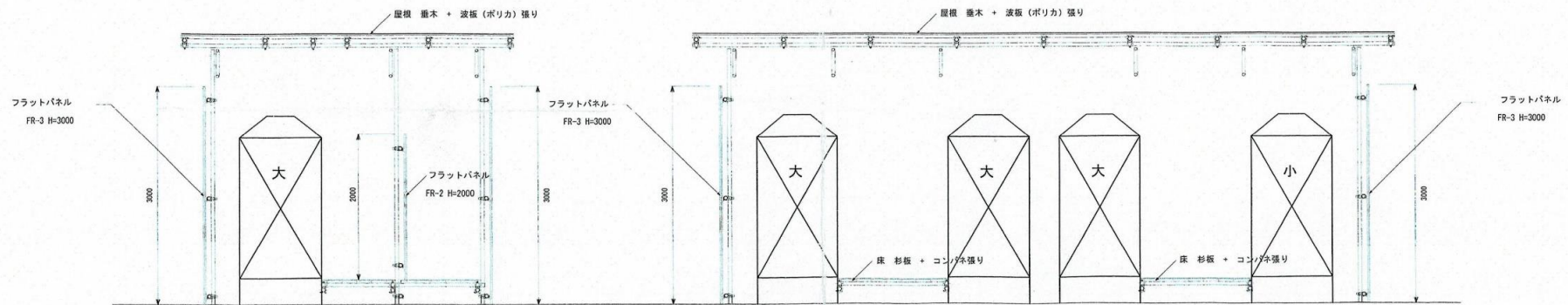
A - A' 断面図
