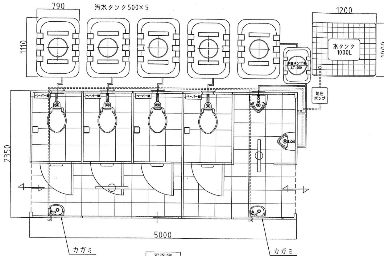
平面図
