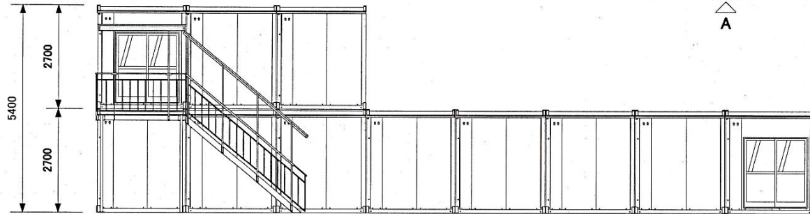
A 立面图
