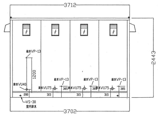
背面図
