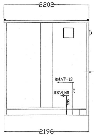
左側面図
