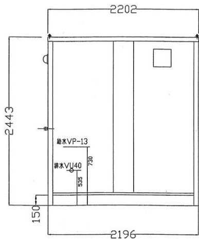
右側面図
