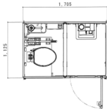
平面図 S=1/30
