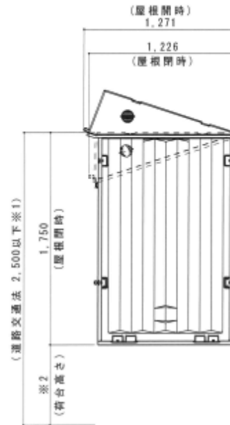
D 立面図 S=1/30
