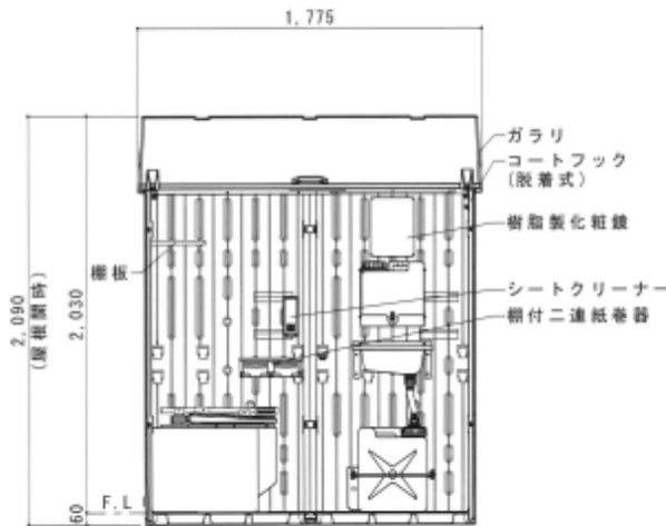
断面図 S=1/30
