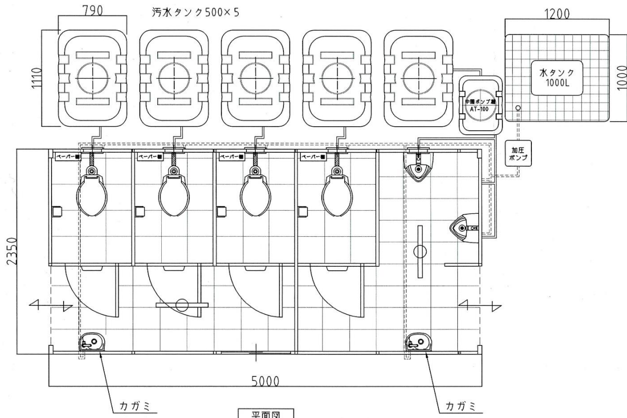
平面図
