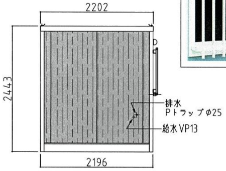
左側面図
