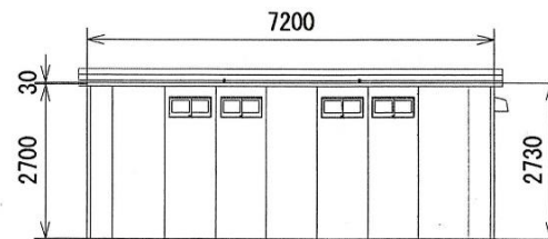
C立面図 S=1:100
