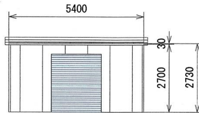
D立面図 S=1:100
