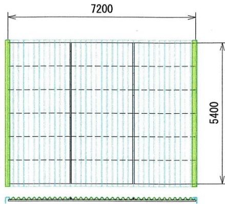
屋根伏図 S=1:100
