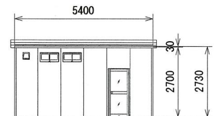
B立面図 S=1:100
