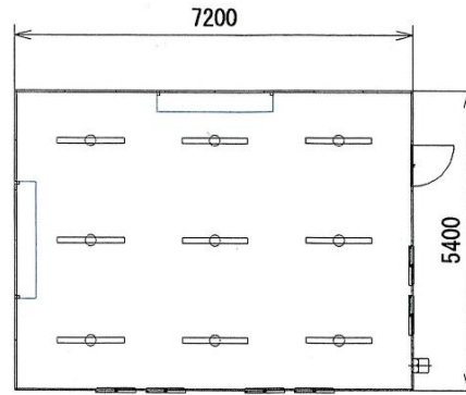
平面図 S=1:100
