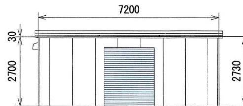
A立面図 S=1:100
