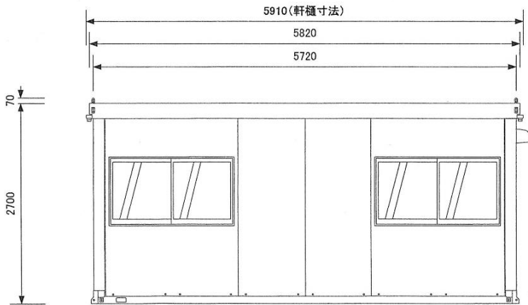
A 立面図
