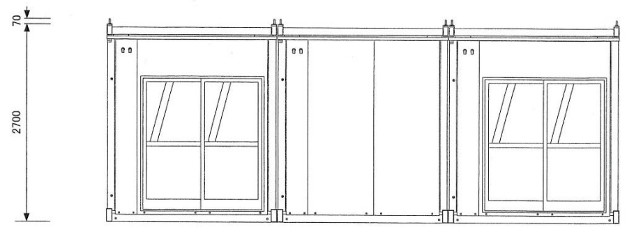
A 立面図
