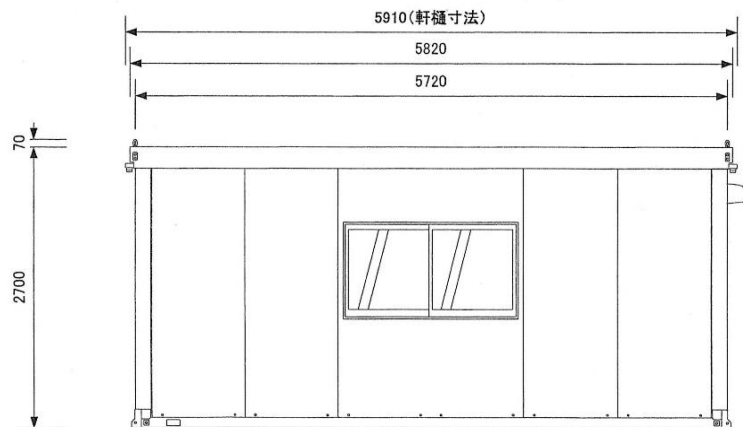
A 立面図
