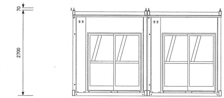
A 立面図
