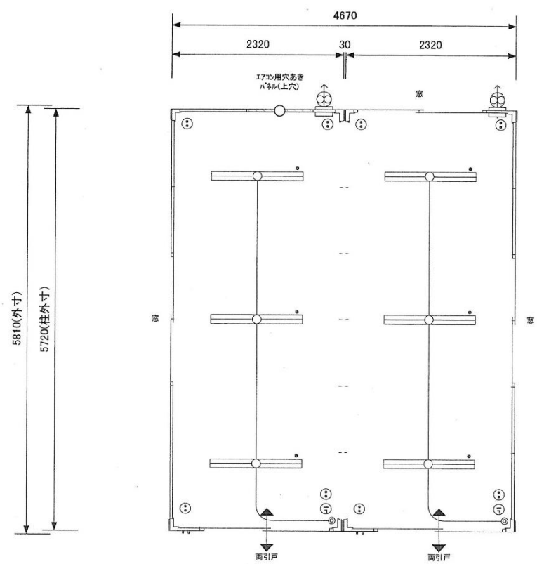
平面図
