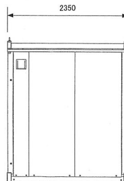
D 立面図
