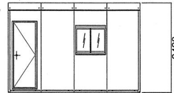
正面図
