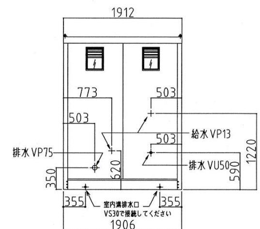
背面図
