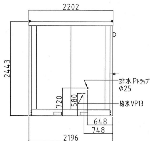
左側面図
