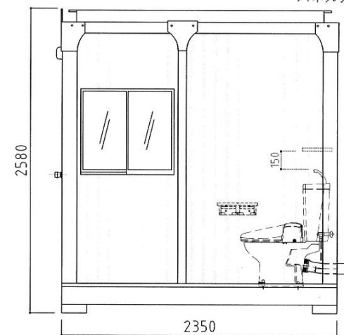
右側面図
