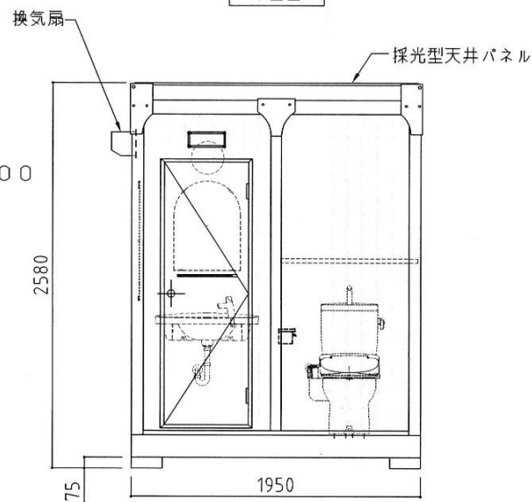
正面図
