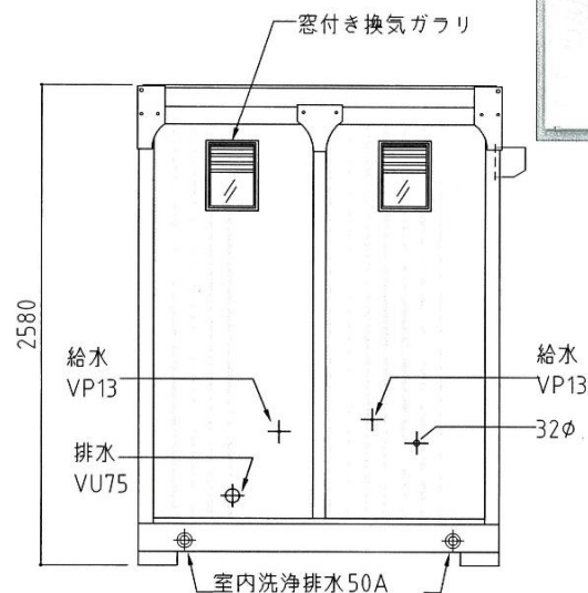
背面図
