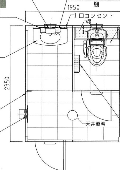
平面図
