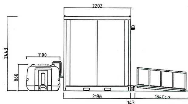
左側面図
