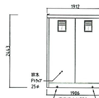
背面図
