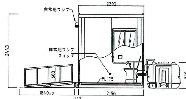
右側面図
