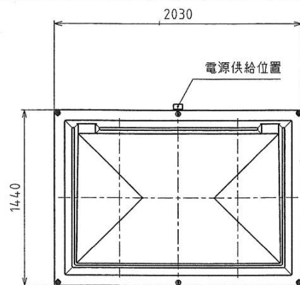
屋根伏図
