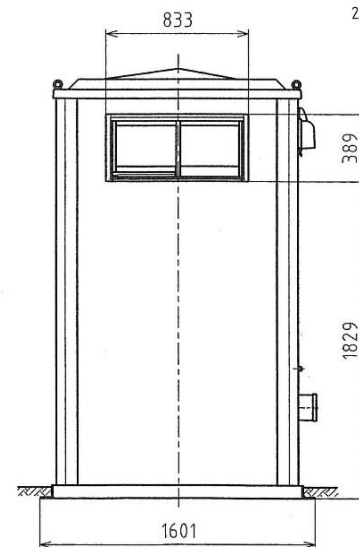
右側面図
