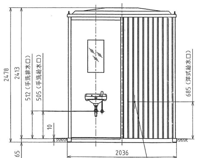
正面図
