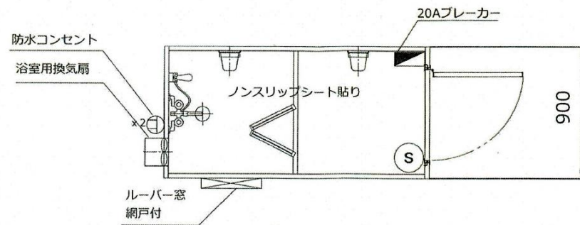
平面図
