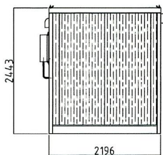
左側面図
