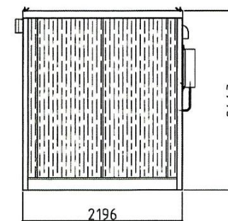
右側面図
