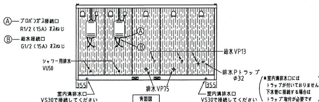
背面図
